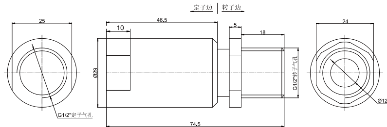
MK14A 尺寸图
