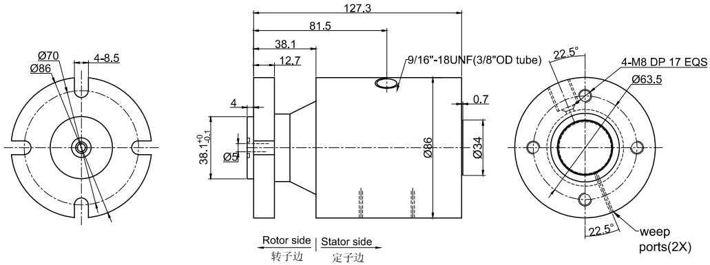
MHPS16 (高压不锈钢旋转接头) 尺寸图
